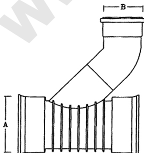
A- مخصوص اتصال لوله‌های دوجداره B- مخصوص لوله تکجداره PVC, PP, PE
