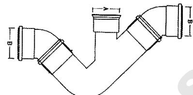
A- مخصوص اتصال لوله‌های دوجداره B- مخصوص لوله تک‌جداره PVC, PP, PE یا تبدیل لوله دوجداره
