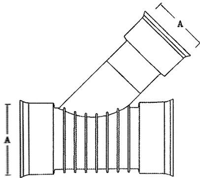
A- مخصوص اتصال لوله‌های دوجداره
