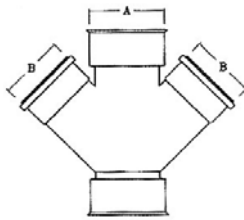
A - مخصوص اتصال لوله‌های دوجداره B - مخصوص لوله تک‌جداره PVC, PP, PE
