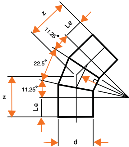
Elbow 45°
